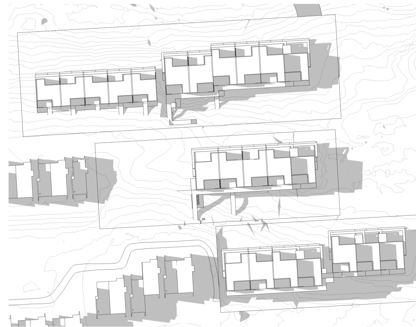
4 SOLSTUDIE_21.JUNI_KL.19 L 1: 1000
