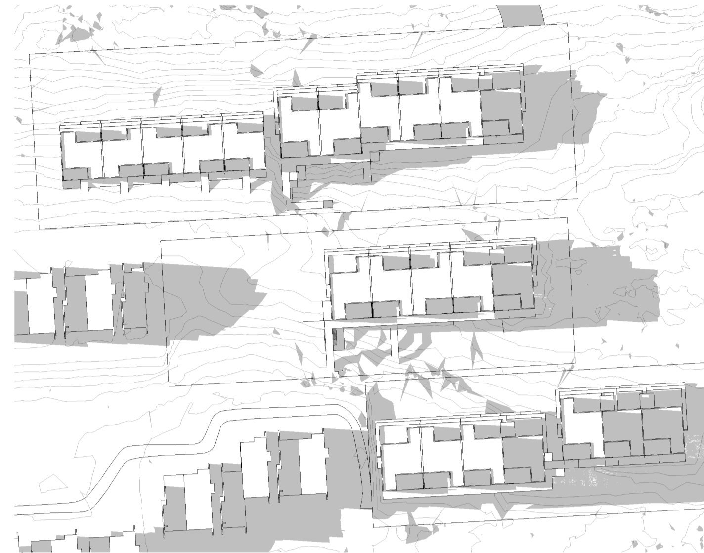
6 SOLSTUDIE_01.MAI_KL.19 L 1: 1000
