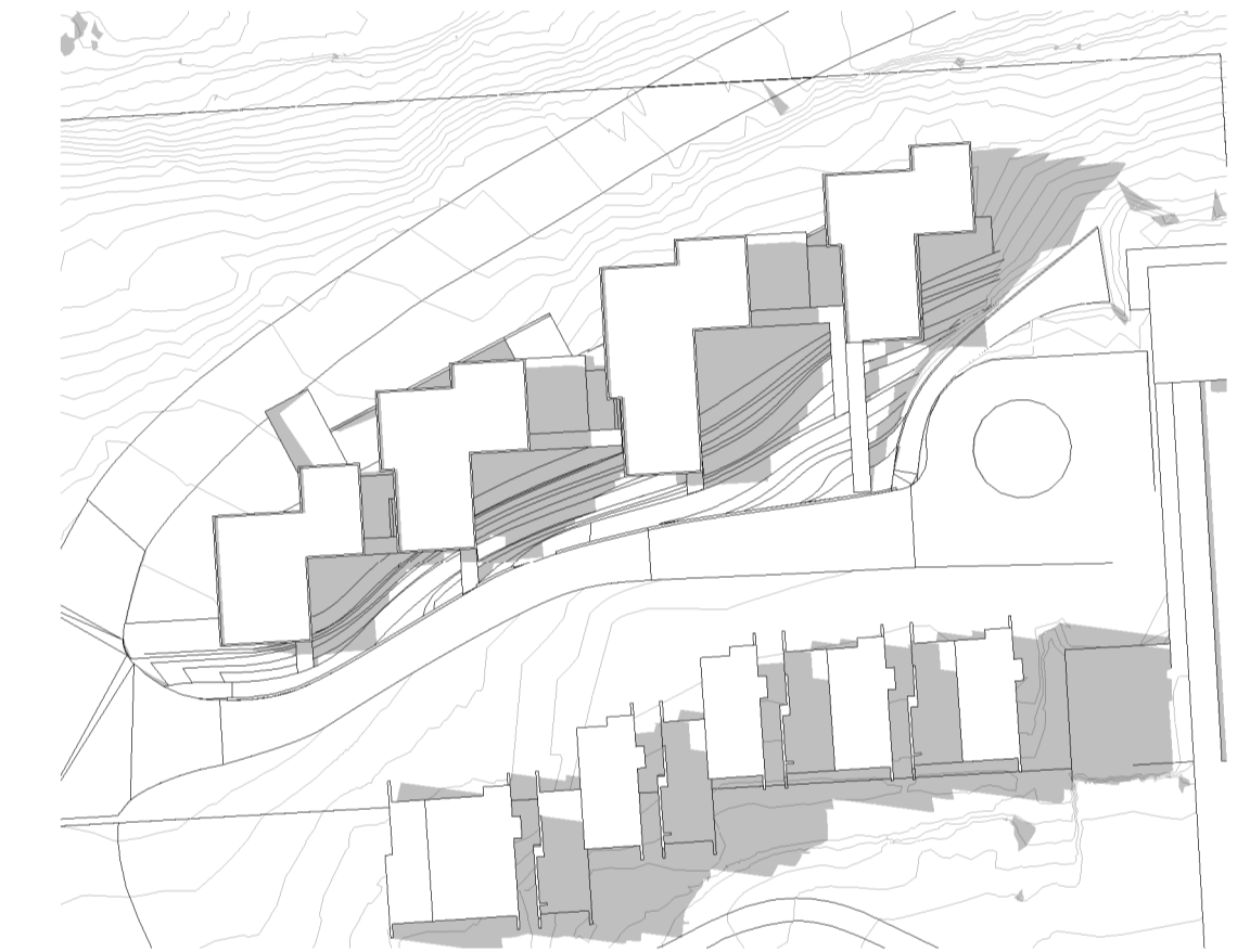
10 SOLSTUDIE_21.JUNI_KL.19 H 1:1000
