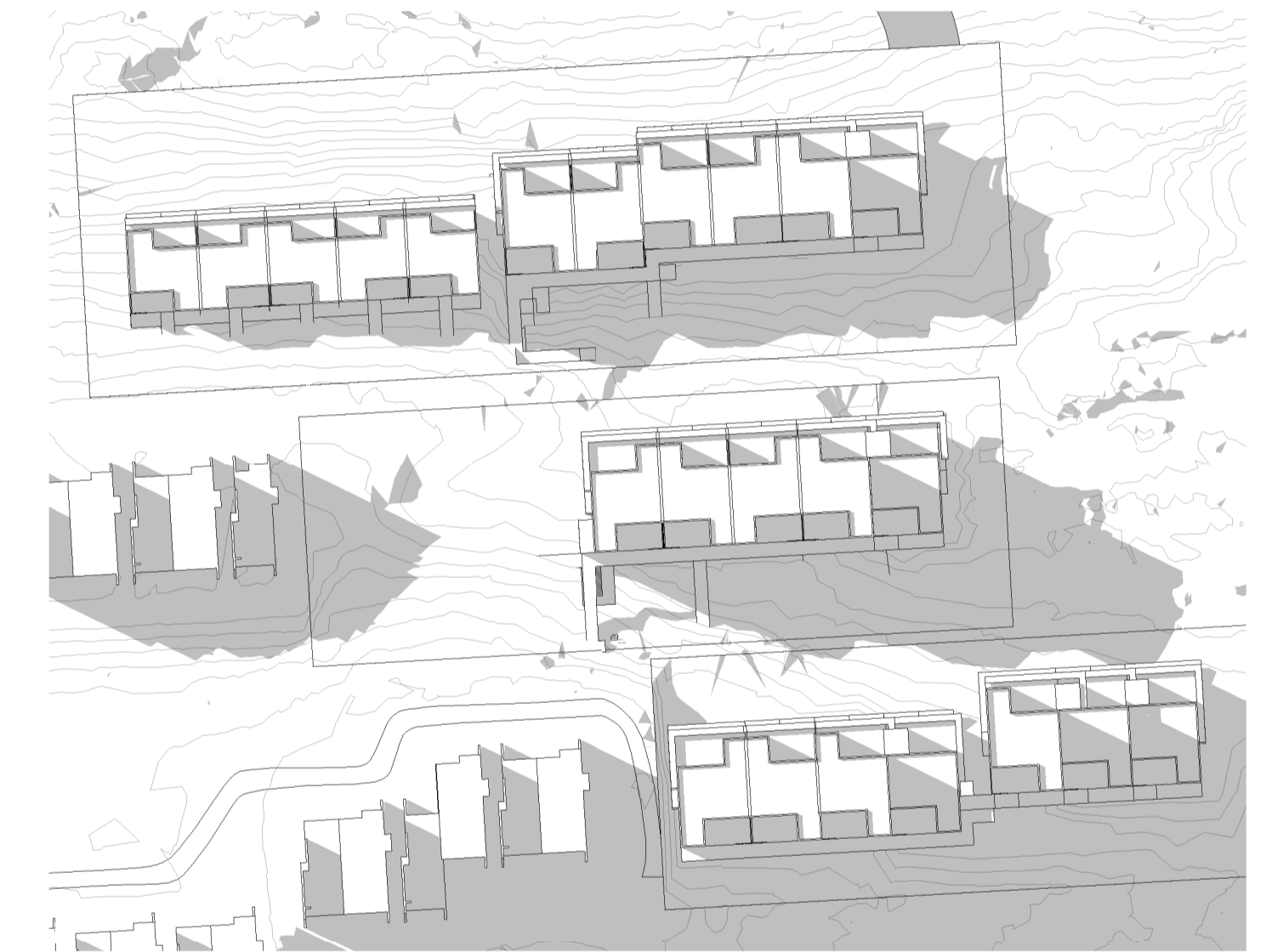
8 SOLSTUDIE_21.JUNI_KL.20.30 L 1: 1000
