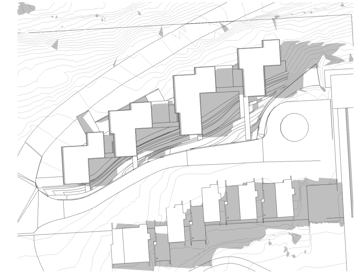
5 SOLSTUDIE_01.MAI_KL.19 H 1:1000
